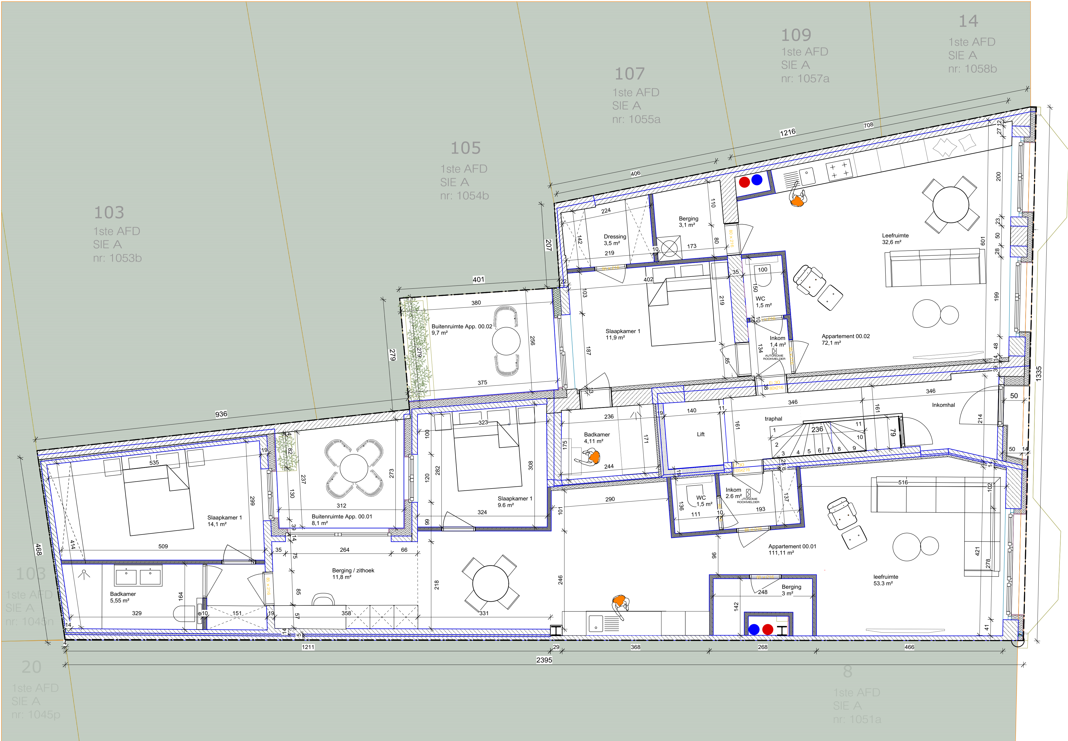
Grondplan Gelijkvloers
